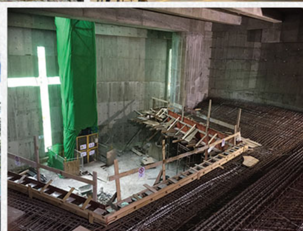
聖堂閣樓工程進行中 — 2017年2月
